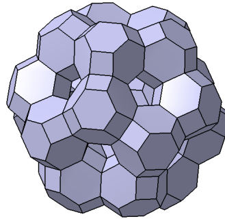
C_{60}(DO_{60})-750
