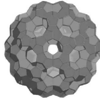
TR(DU(C_{60}(DO_{60})750)662)-5040
